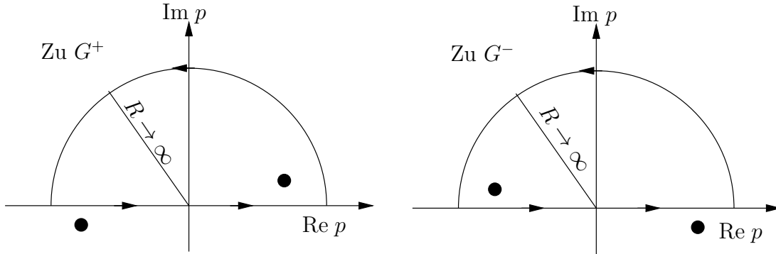
Abbildung 2: Zur Berechnung der freien Greenfunktionen
