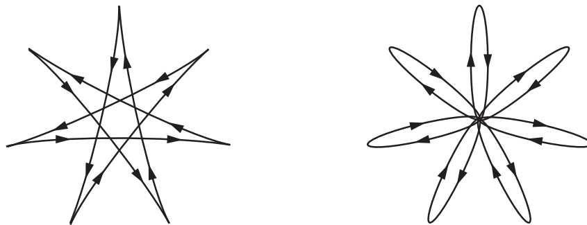
Abbildung 1: Zu Aufgabe 11: Bahnen der Projektion eines Pendels auf der rotierenden Erde für die Anfangsbedingungen (i) (links) und (ii) (rechts). Zur Veranschaulichung wurden \omega_0 und \omega in einem unrealistischen Verhältnis zueinander gewählt (vgl. Aufgabenteil (c)).
